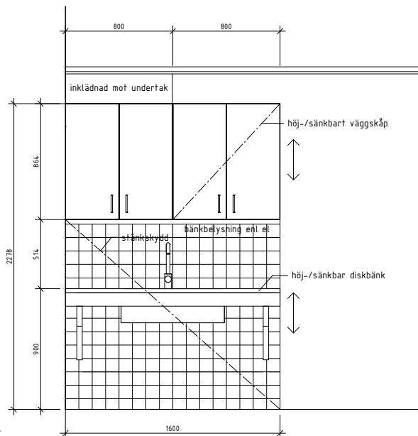
GEMENSAMT KÖK - VY 2 SKÅPINREDNING TYP 2
