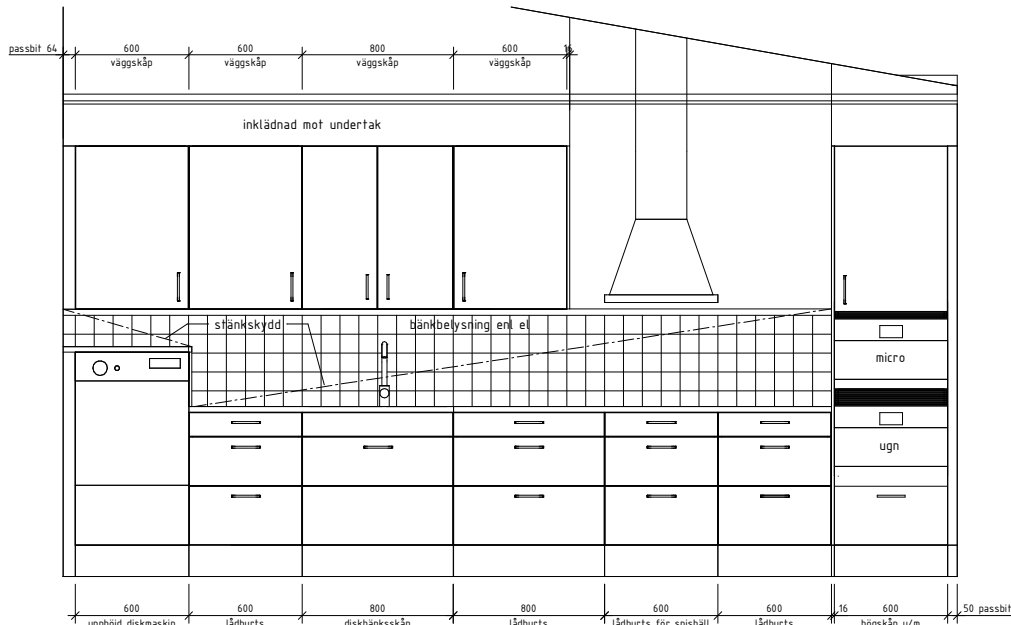
GEMENSAMT KÖK - VY 1
